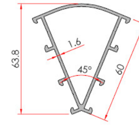
135° Corner Adapter 135° Köşe Dönüş Adaptörü
