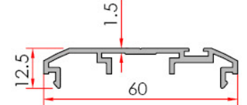
Swing Door Adapter (Vent) Çarpma Kapı Adaptörü (Kanat)
