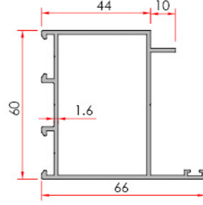
Vent Kanat
