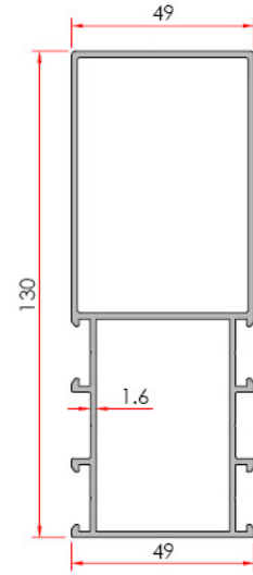
Reinforced Meeting Rail Takviyeli Orta Kayıt
