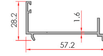
Vent Adapter Kanat Adaptörü
