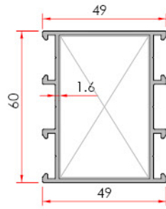
Frame Kasa
