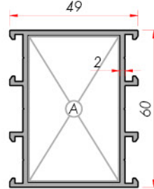
Frame Kasa
