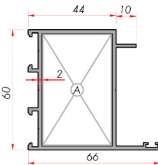
Vent Kanat
