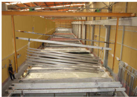
Anodizing Line / Eloksal Hattı
