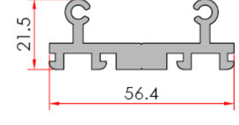
Connection Bağlantı
