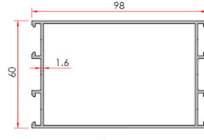
Vent Kanat
