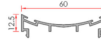
Swing Door Adapter (Frame) Çarpma Kapı Adaptörü (Kasa)
