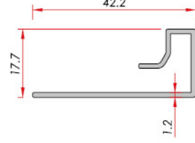
Dilatation Profile Dilatasyon Kapak
