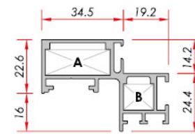
Bonding Lath Narrow Glass Panel (Vent) Bonding Çıtalı Dar Cam Paneli (Kanat)
