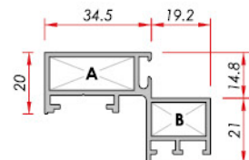
Narrow Glass Panel (Vent) Dar Cam Paneli (Kanat)
