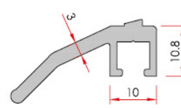
Inside Corner Turn Clip İç Köşe Dönüş Klipsi
