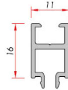
Single Glass Bead Tek Cam Çıtası
