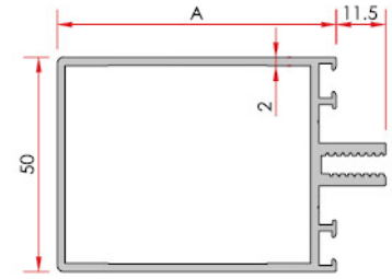
Transom Profiles Transom Profilleri
