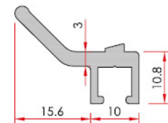
Outside Corner Turn Clip Dış Köşe Dönüş Klipsi
