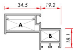
Glazing Panel (Vent) Cam Paneli (Kanat)
