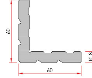
Corner Cleat Köşe Takoğu
