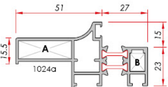
Insulated Glazing Panel (Sash) Yalıtımlı Cam Paneli (Kanat)
