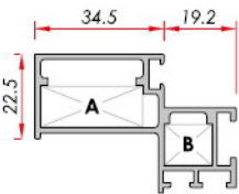
Glazing Panel (Vent) Cam Paneli (Kanat)
