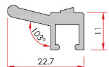
Angular Clip Açılı Klips
