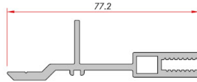
Half Mullion Adapter Yarım Mulyon Adaptörü
