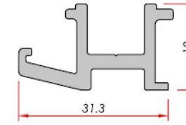
Panel Assembling Wedge Kaset Montaj Takozu
